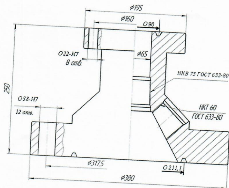
Схема планшайбы
