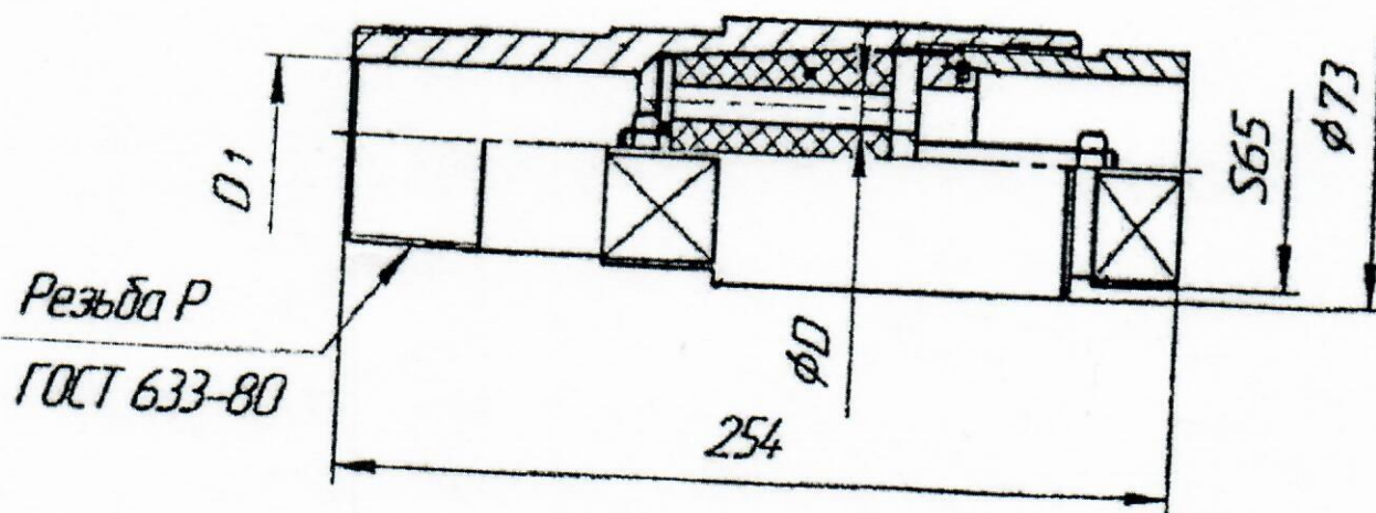
Кабельный ввод КВ-3-60х35-1
