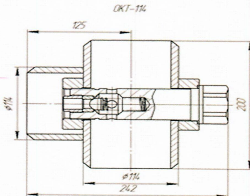
Эскиз обратного клапана
