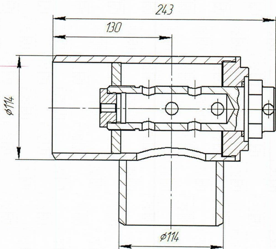
Эскиз штуцерной камеры
