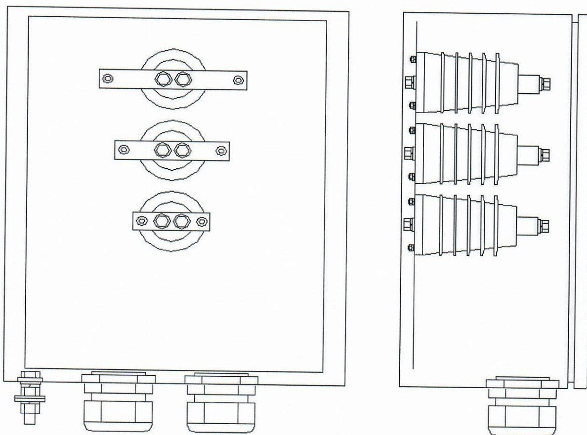
Схема клемной коробки
