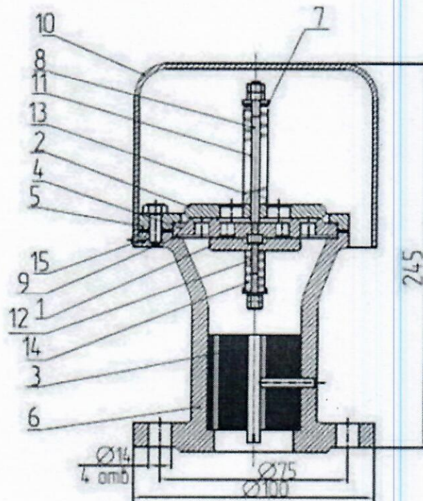
Эскиз КДМ-50М
