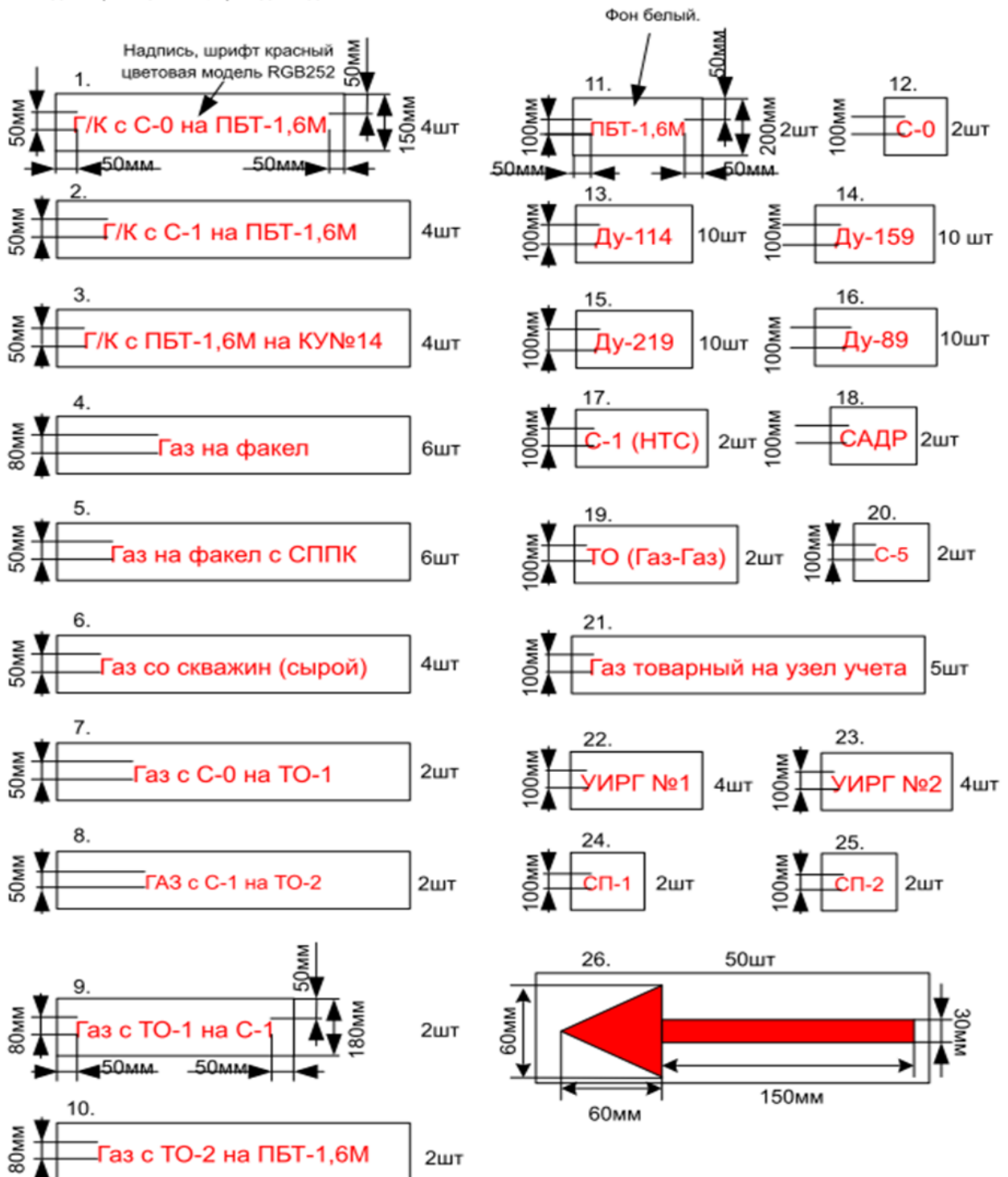
Схема №1 Наклейка для маркировки оборудования. Атмосферостойкие (стойкие к ультрафиолету), водонепроницаемые, пригодные для мытья.
