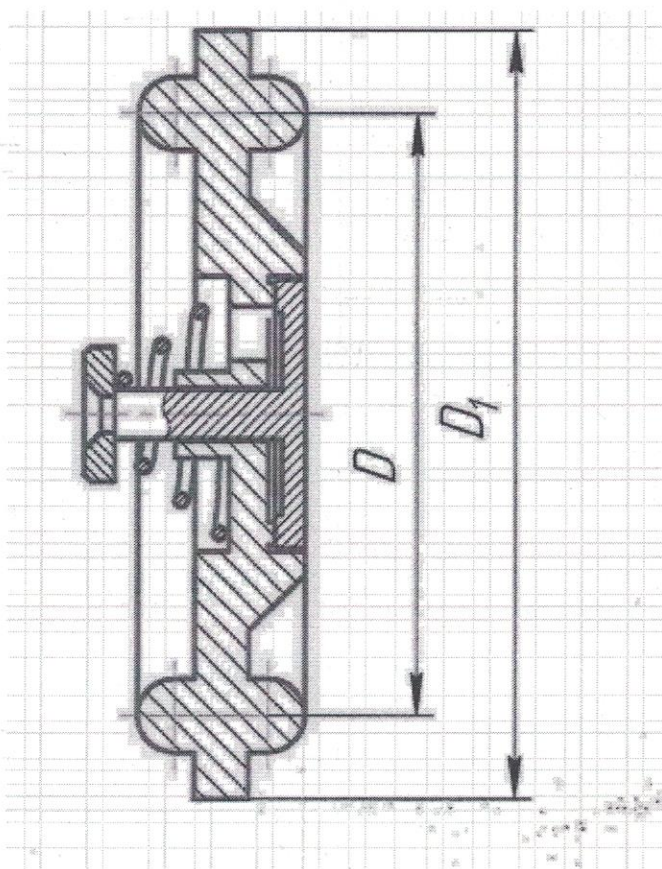
Эскиз обратного клапана
