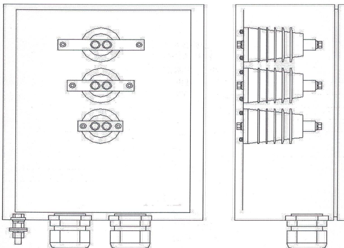
Схема ШСВГ
