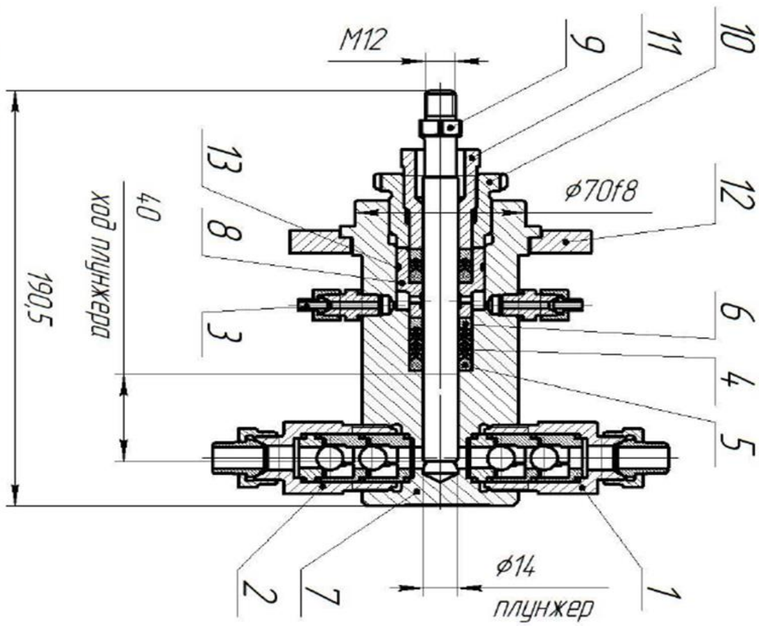
Рисунок 2 - Гидроцилиндр
