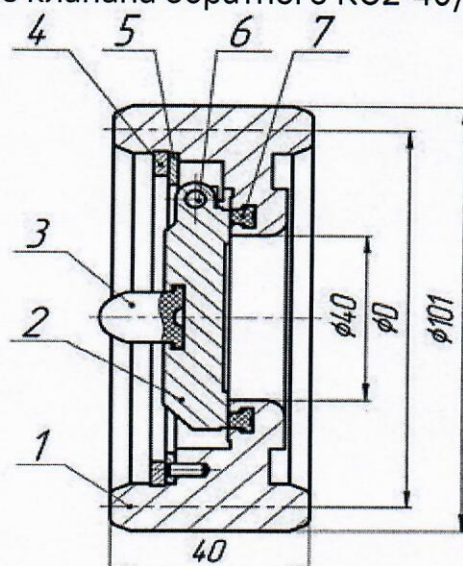
Эскиз клапана обратного КО2-40/65х35
