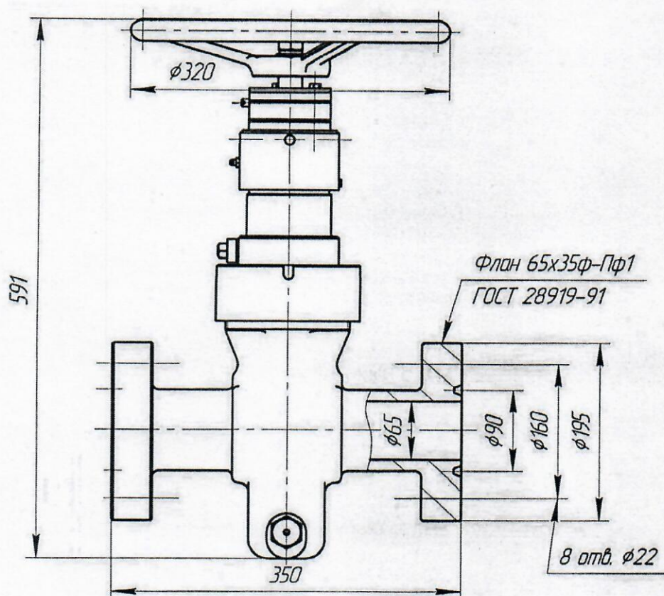
Схема задвижки с КМЧ
