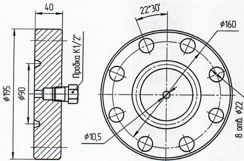
Схема глухого фланца
