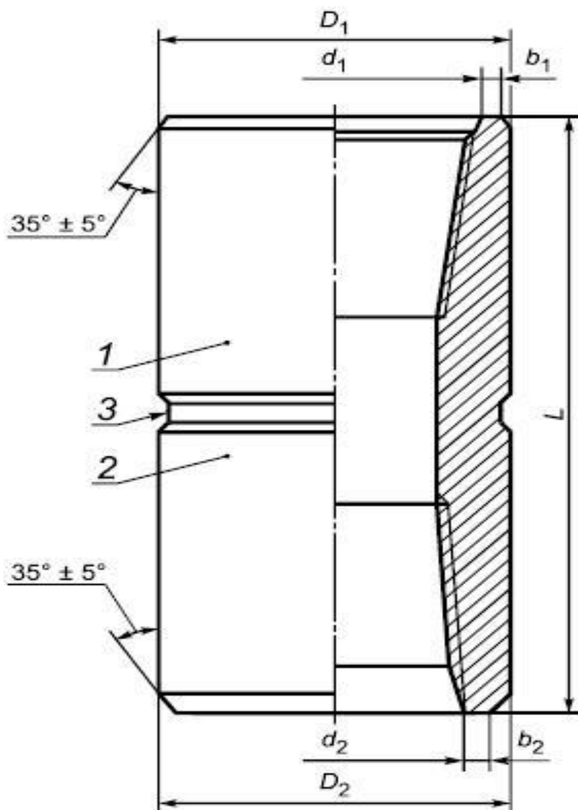
Схема муфтового переводника.
