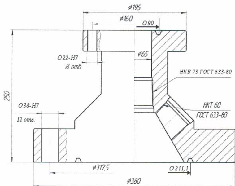
Схема планшайбы
