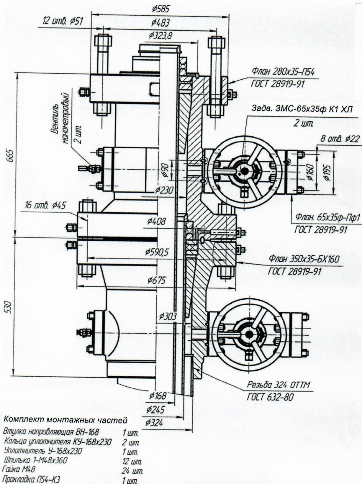
Схема ОКК-2
